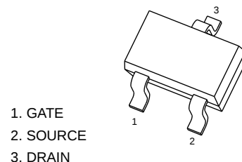
SOT-323
